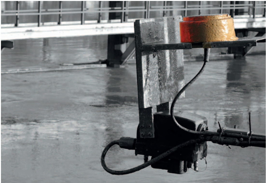
Split-beam-Schallgeber eines wissenschaftlichen Echolots. Mit Blick auf die Fragestellung sind Montage und Anordnung der Technik sowie deren Wartung entscheidend für die Qualität der Datenerfassung, besonders in Flüssen mit hohen Sedimentfrachten.
